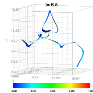
図1 螺旋状の流れによって、もともとまっすぐだった磁力線がどのように変形するかを計算した結果。磁場生成の基礎的なメカニズムを解き明かすための研究より
