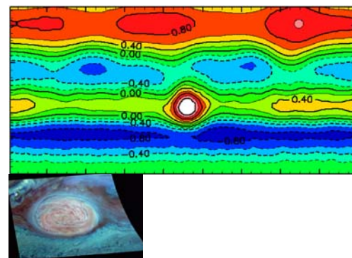
図6. 地球の海の数値モデルに基づいて作成した数値モデルの中に生まれた大規模な渦。木星の大赤斑(下)と構造や振る舞いが似ている。
