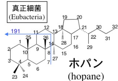
図3 真核生物と真正細菌にそれぞれ特有なステランとホパンの化学構造
