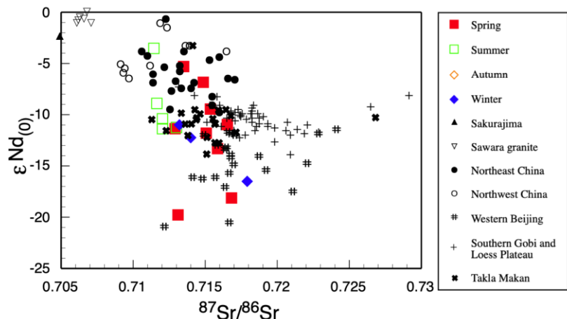
脊振山頂で採取した風送塵(黄砂など)の Sr・Nd 同位体組成と砂漠や火山灰の組成の比較。組成の違いから、風送塵の起源と季節変化を探ることができる。
