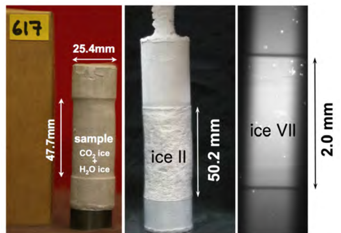
図5 惑星氷の高压下での変形実験
