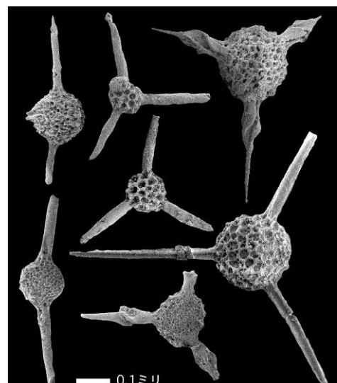
図2 後期三畳紀の放散虫化石種の一例。
