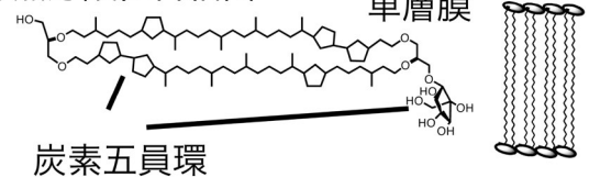
図4 好熱好酸性古細菌の培養と膜脂質
