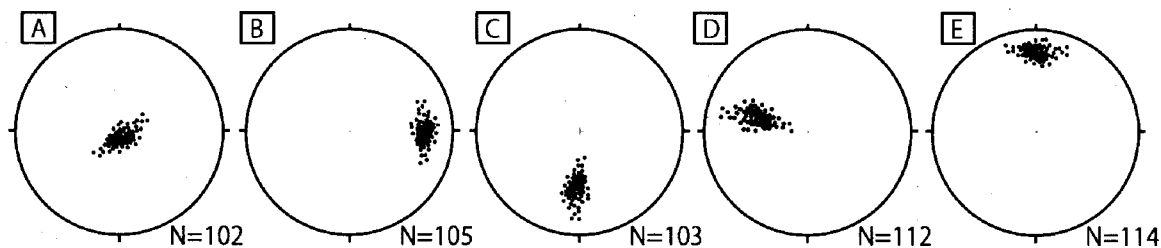
図 3 粘板岩中にみられる劈開のステレオ投影図 (下半球投影)
